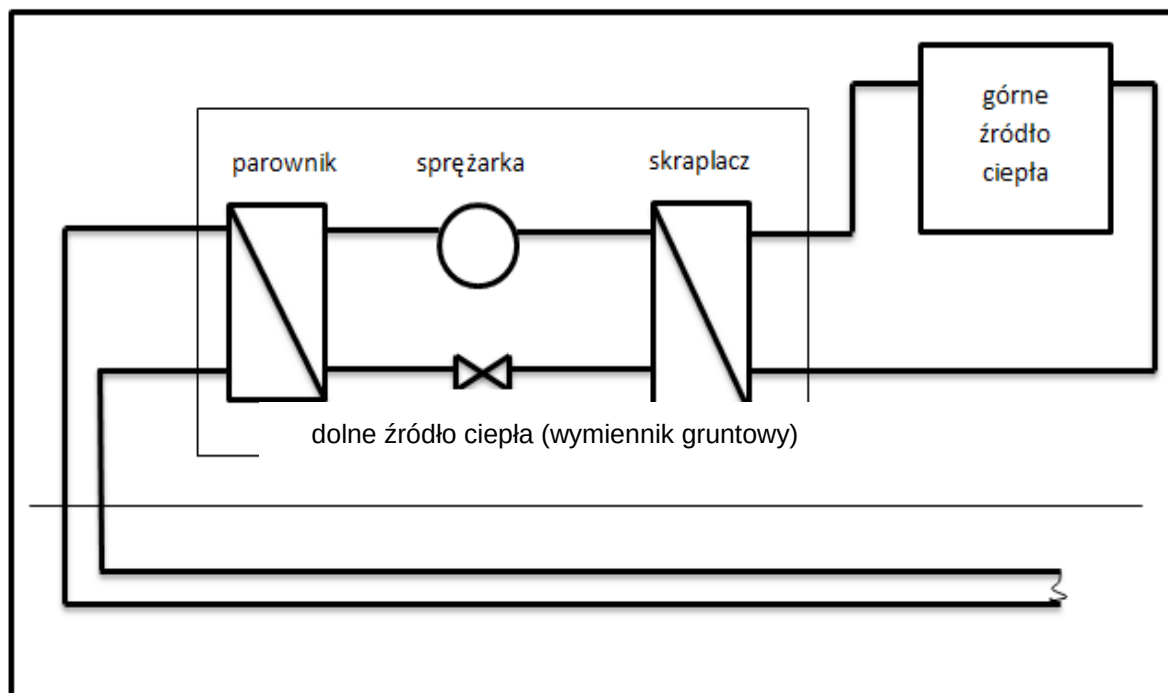
Rysunek 32. Schemat działania sprężarkowych pomp ciepła, www.muratorplus.pl .
