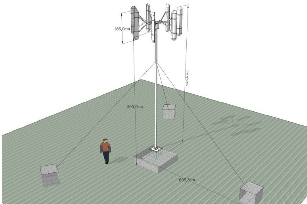
Rysunek 33. Parametry techniczne mikroturbiny wiatrowej, http://generatory-wiatrowe.pl/?page_id=21 .
